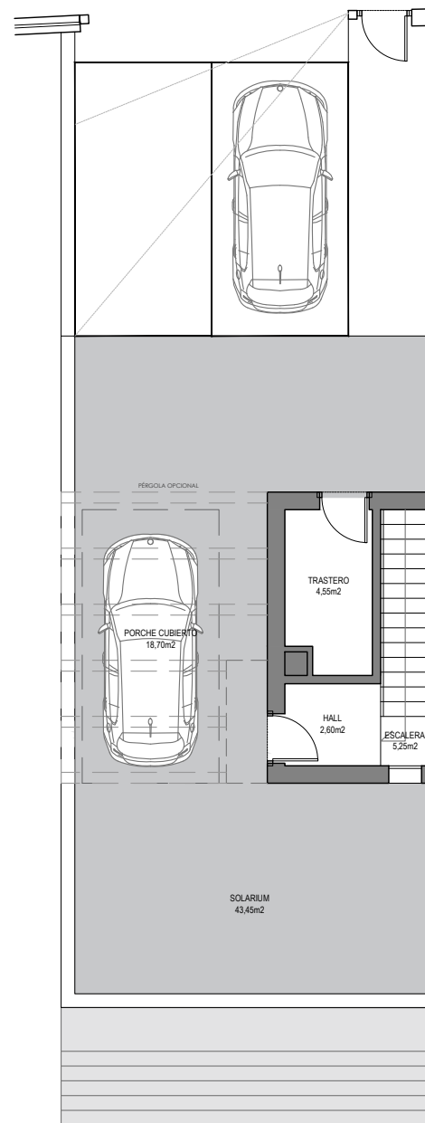
PLANTA SOLARIUM
