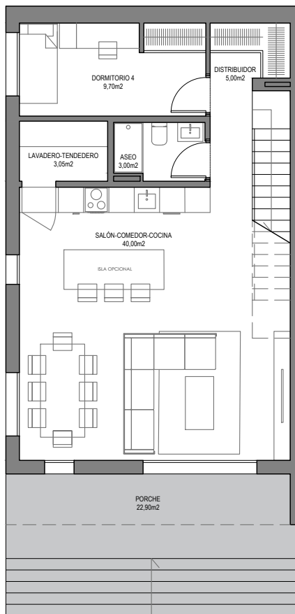
PLANTA BAJA
