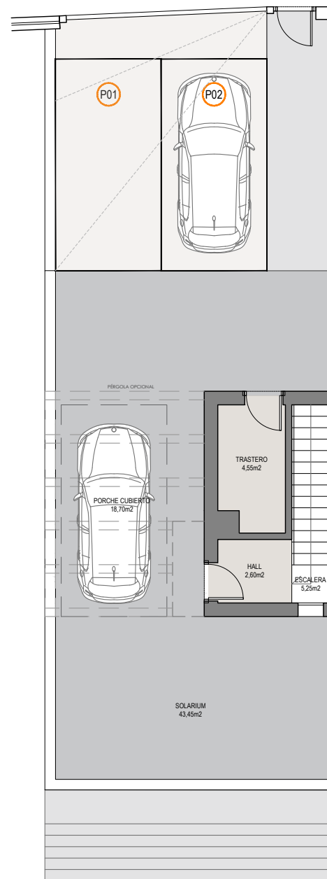
PLANTA SOLARIUM
