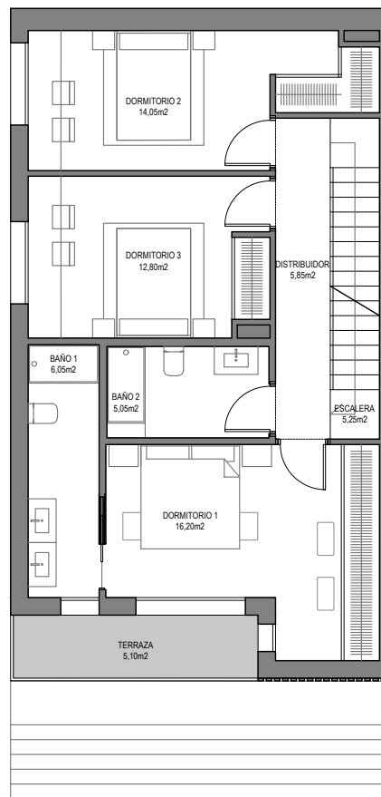
PLANTA PRIMERA
