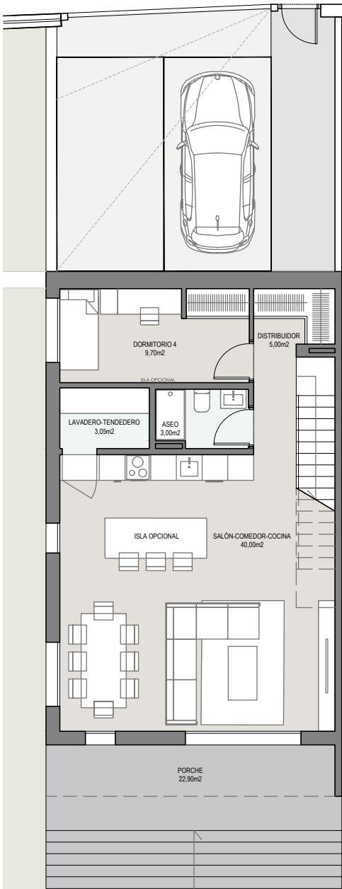
PLANTA BAJA
