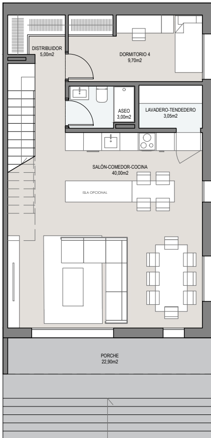
PLANTA BAJA
