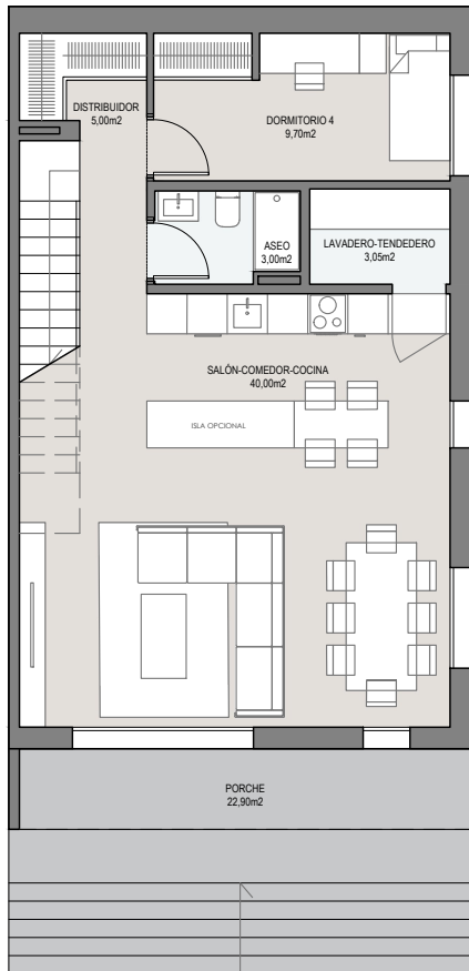
PLANTA BAJA
