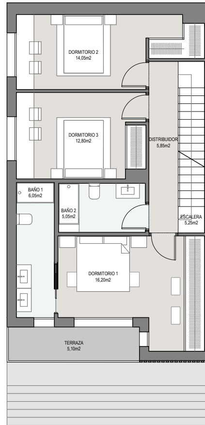
PLANTA PRIMERA
