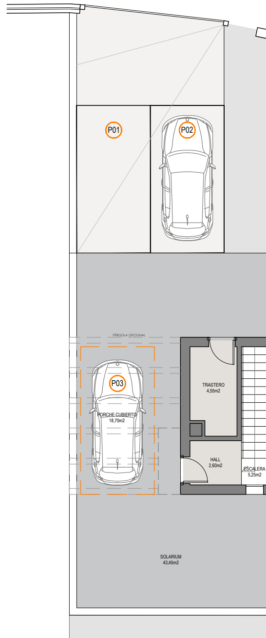
PLANTA SOLARIUM
