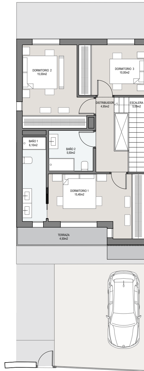
PLANTA PRIMERA
