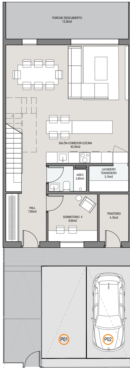
PLANTA BAJA
