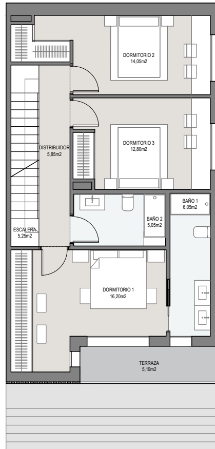
PLANTA PRIMERA
