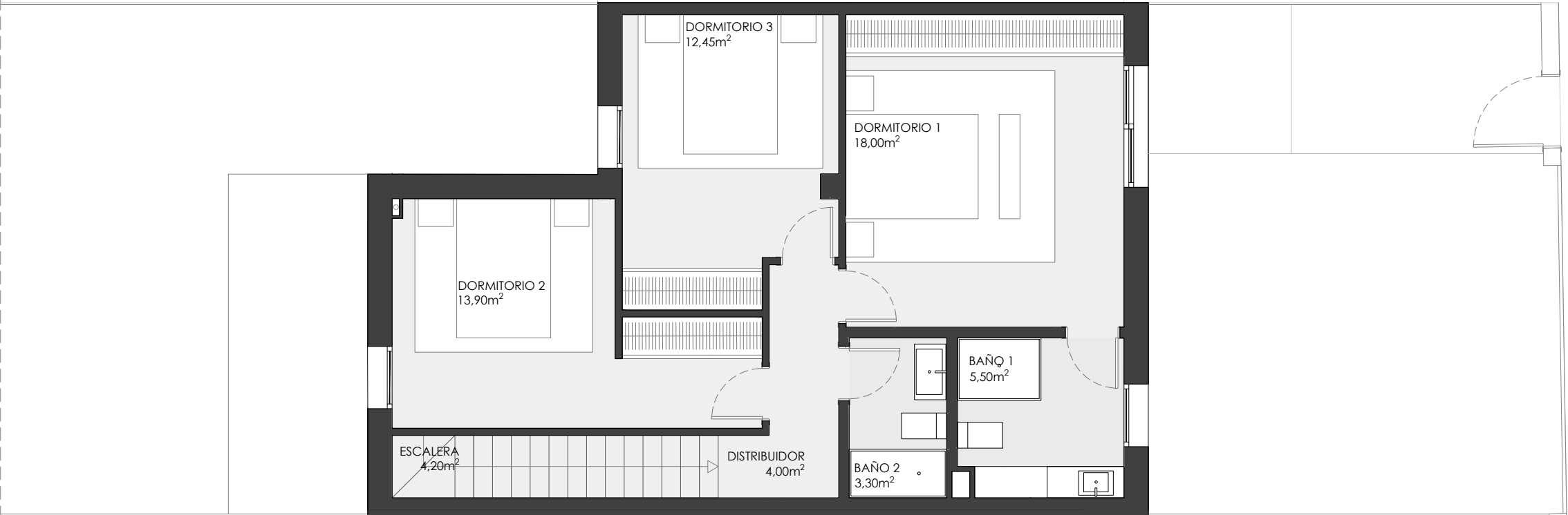
PLANTA PRIMERA
