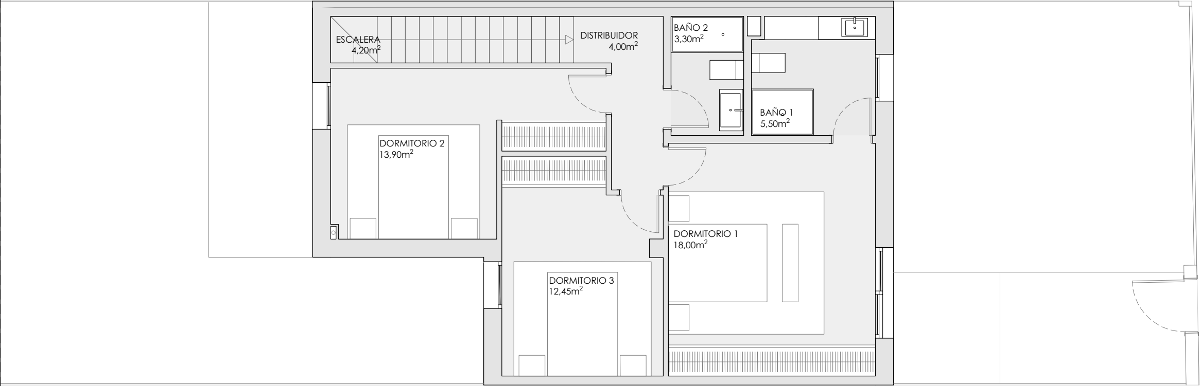
PLANTA PRIMERA
