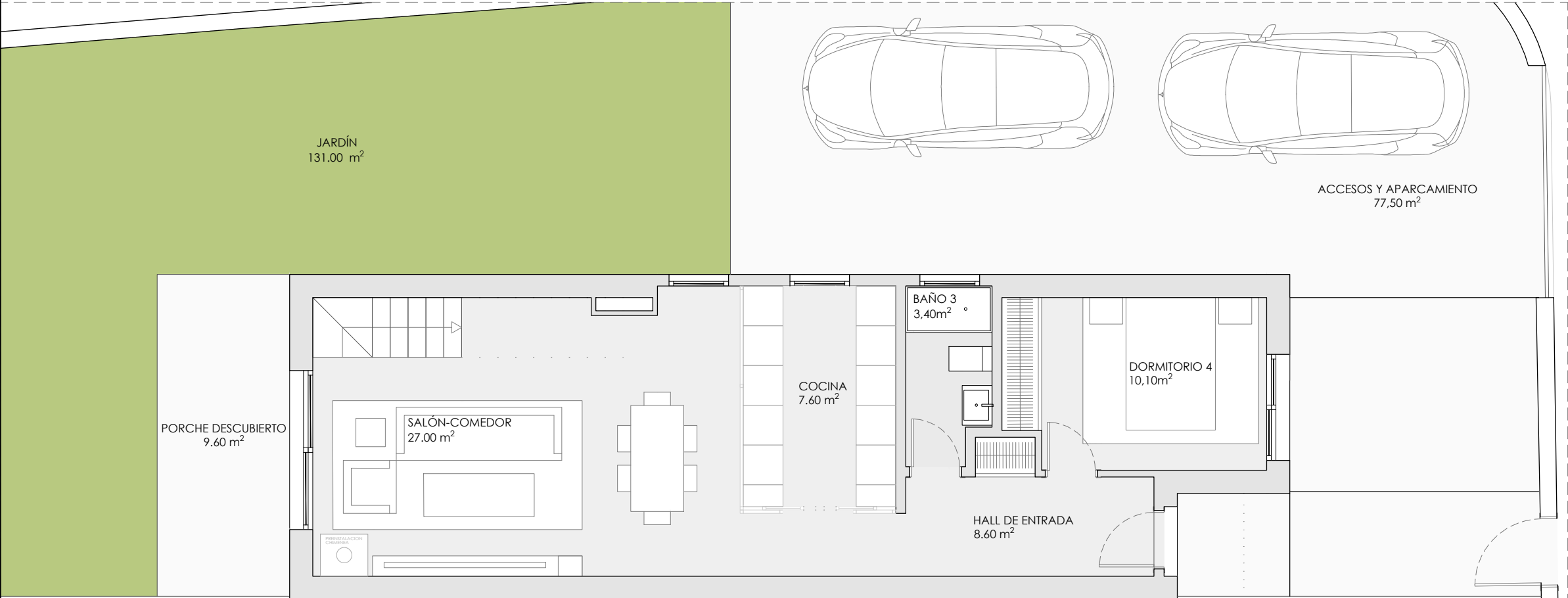
PLANTA BAJA
