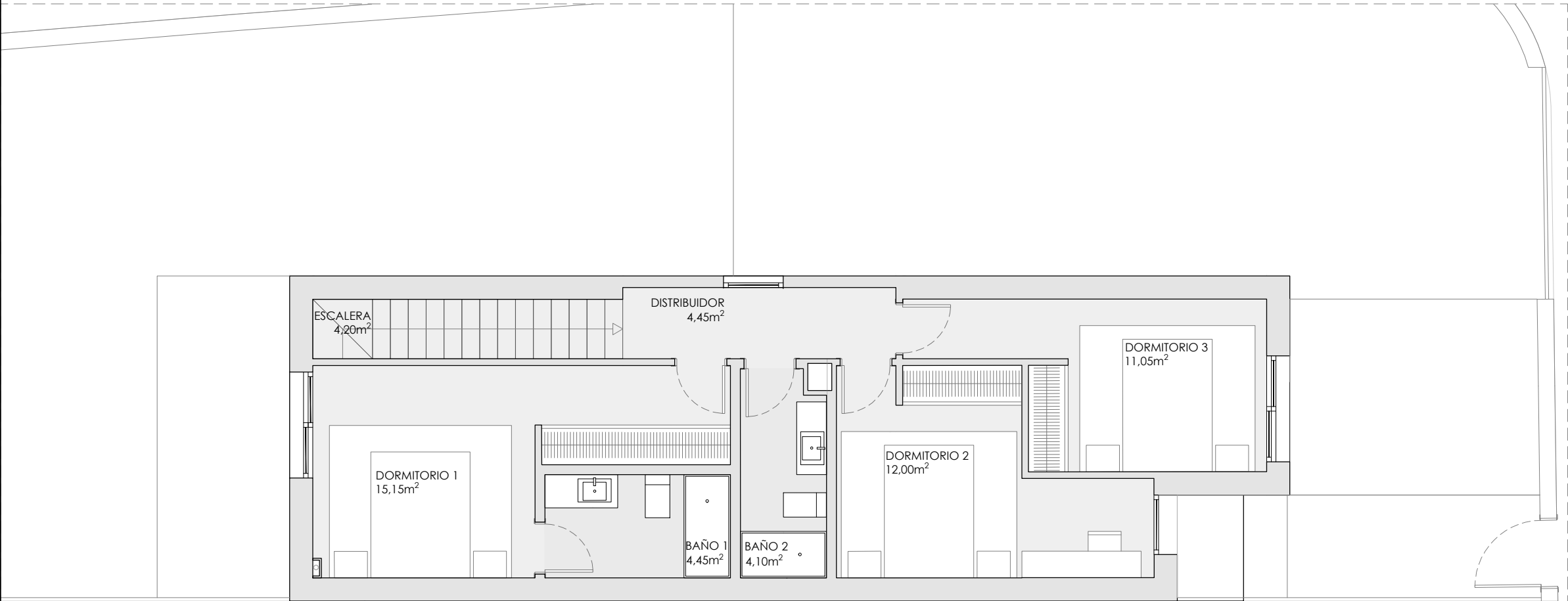
PLANTA PRIMERA
